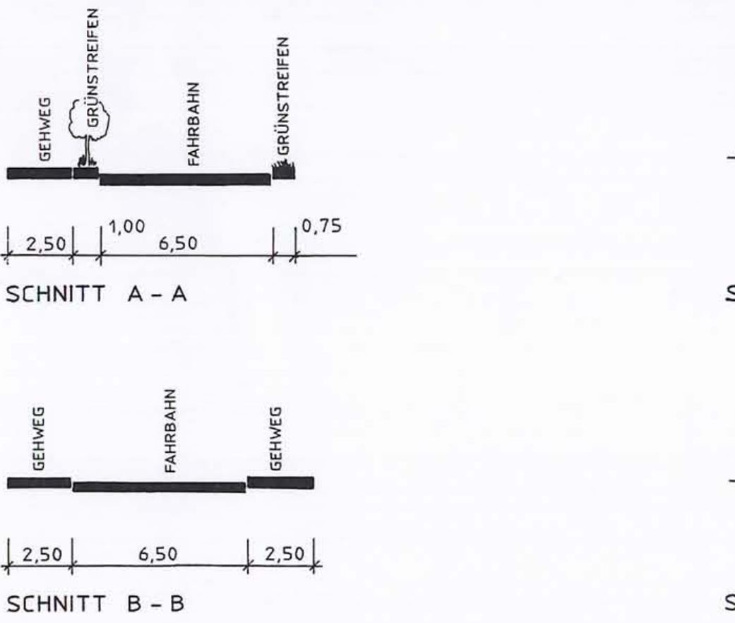
STRASSEN- UND WEGEQUERSCHNITTE M 1:200
