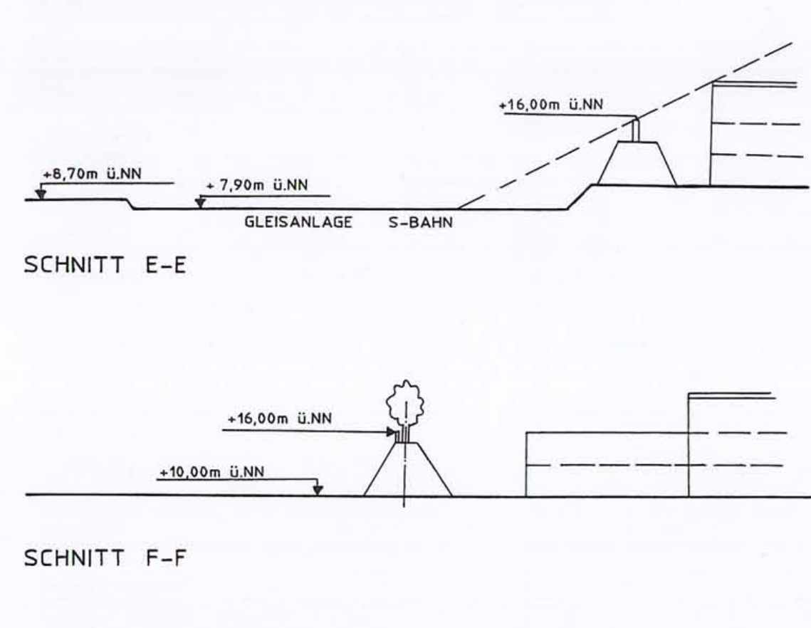
QUERSCHNITTE LÄRMSCHUTZ M 1:500
